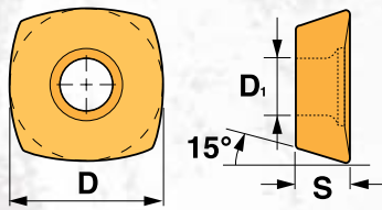
Chipbreaker Style
