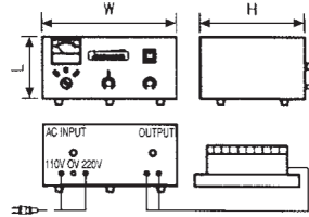
GÜÇ KAYNAĞI
